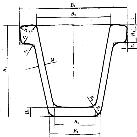
图 1 18U 截面图
