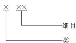
图 1 代码结构图
