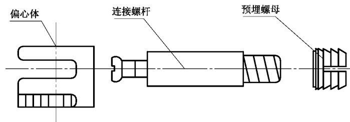
图 1 三合一偏心连接件
