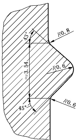
图 1 铣刀轮廓
