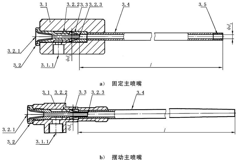
图1 主喷嘴
