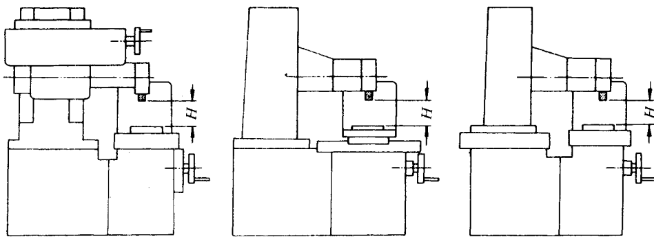
型式 III (立柱移动式)
