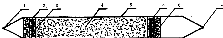
图 1 氨气检测管示意图
