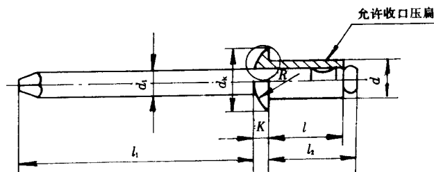
用板材制造的型式
