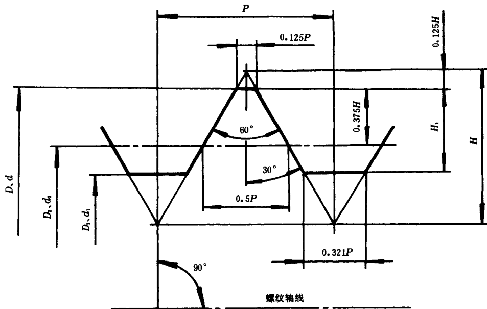
图 1 基本牙型
