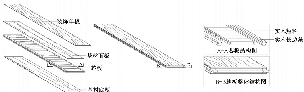
图1 框架式实木复合地板示意图
