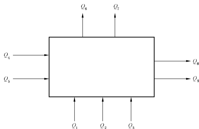
图 1 筛选、CEHP 四段漂白系统能量平衡方框图
