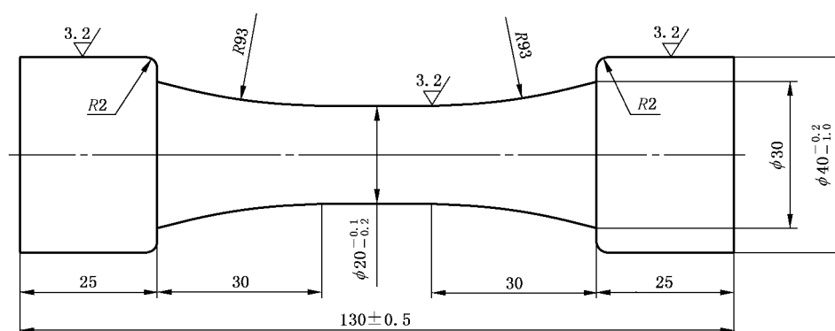
图 1 石墨块材抗拉试样
