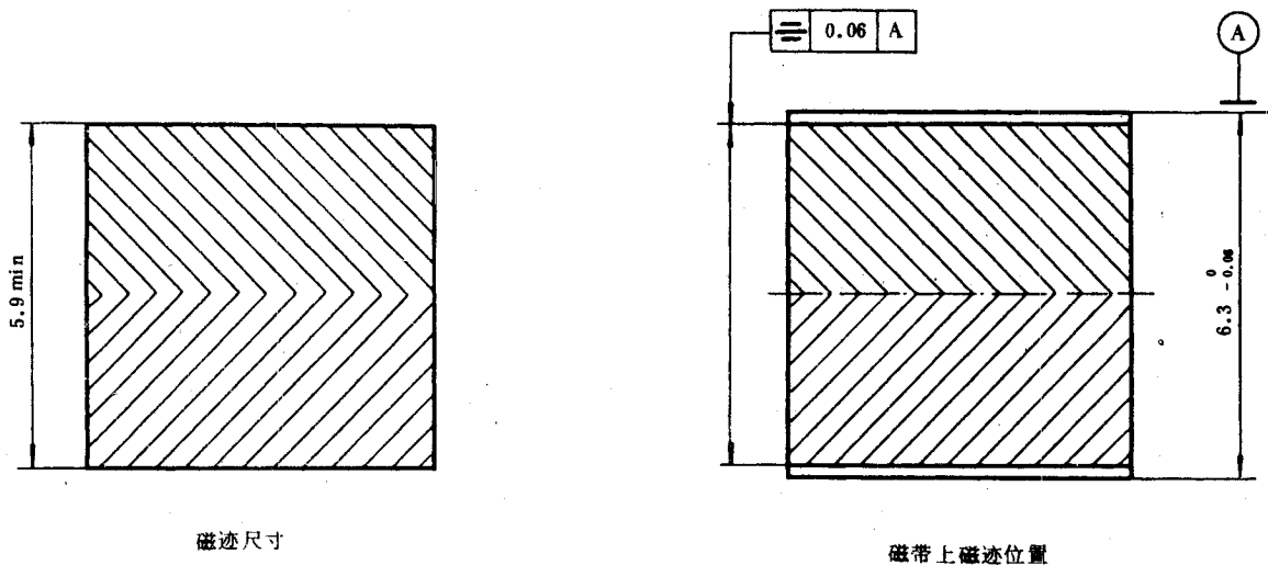
图1 盘式录音机单迹、单道、单向、单道声情况的磁迹形位
