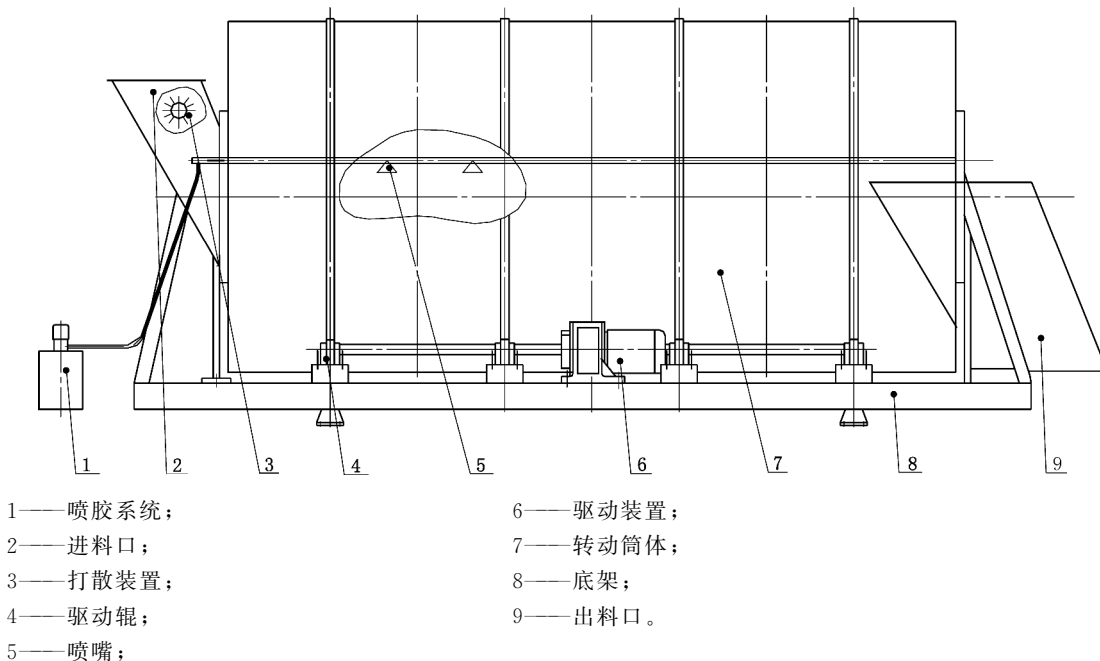
图1 拌胶机结构简图
