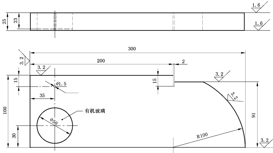
图1 尺寸
