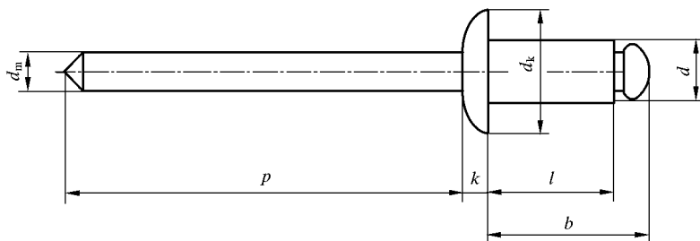
图 1 铆钉尺寸
