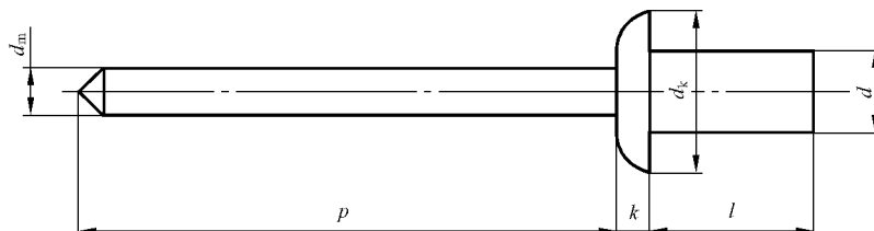
图 1 铆钉尺寸
