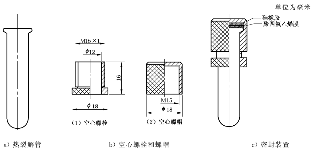
图 1 热裂解管及密封装置
