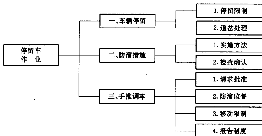
图1 铁路调车停留车作业程序图
