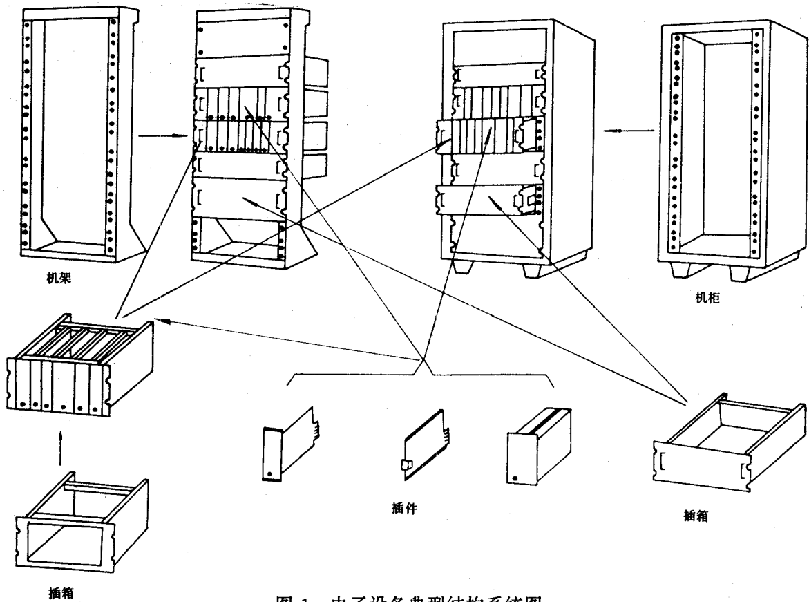
图 1 电子设备典型结构系统图
