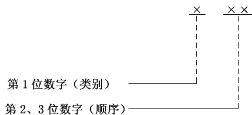
图 1 代码结构图
