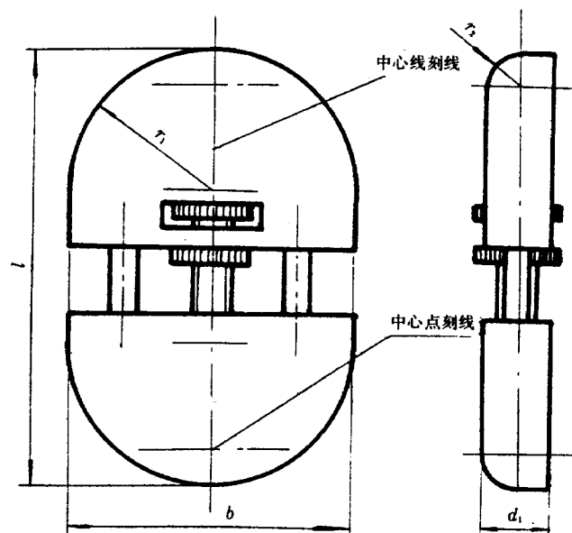
图 1 链窝量规
