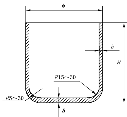
图 1 钨坩埚形状
