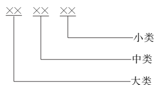
图 1 代码结构图
