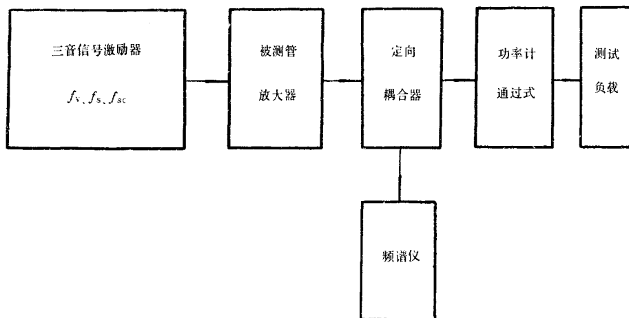
图1 三音互调失真测试方框图
