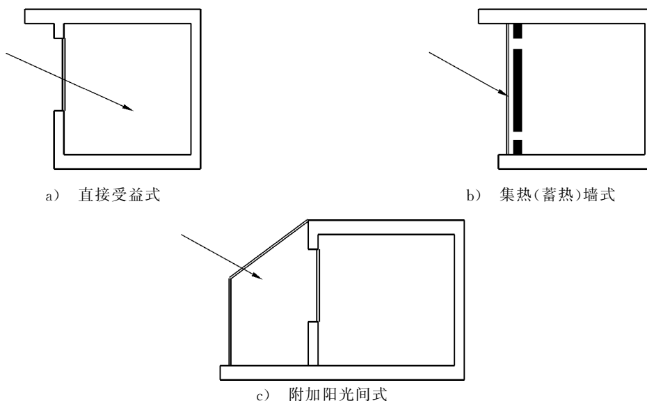
图 1 被动式太阳房的三种形式
