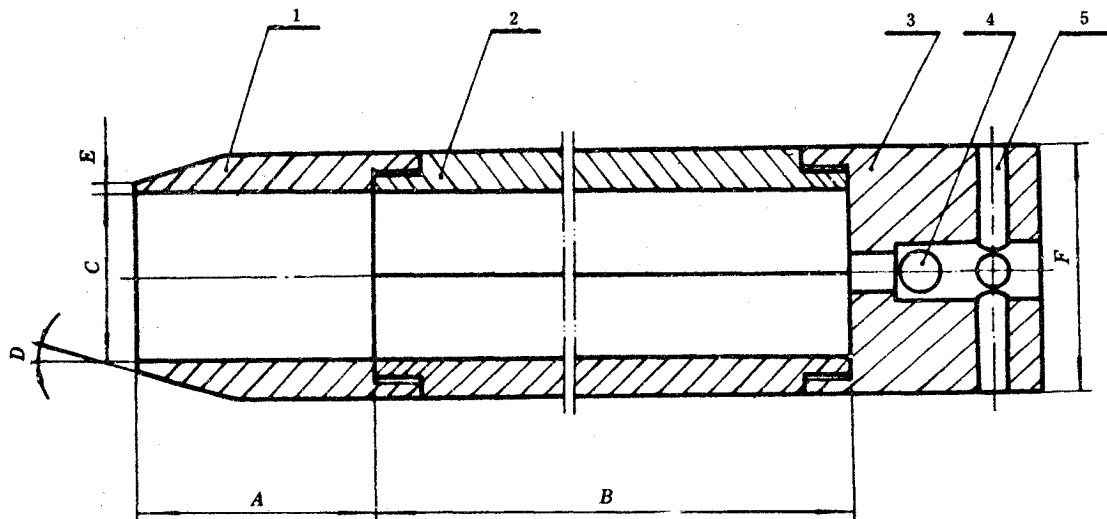
标准贯入器示意图
