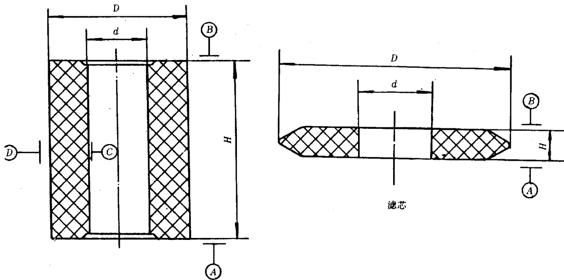
图 1 滤芯
