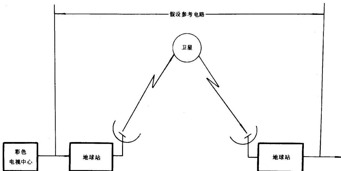
图1 卫星电视/调频假设参考电路
