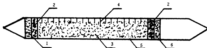
图 1 比长式氨气检测管示意图
