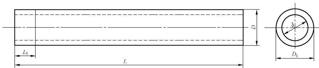
图 1 SiSiC-Rw 型
